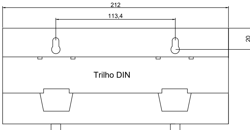
Vista inferior
