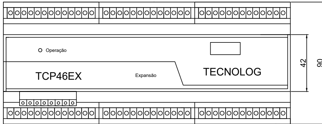
Vista superior
