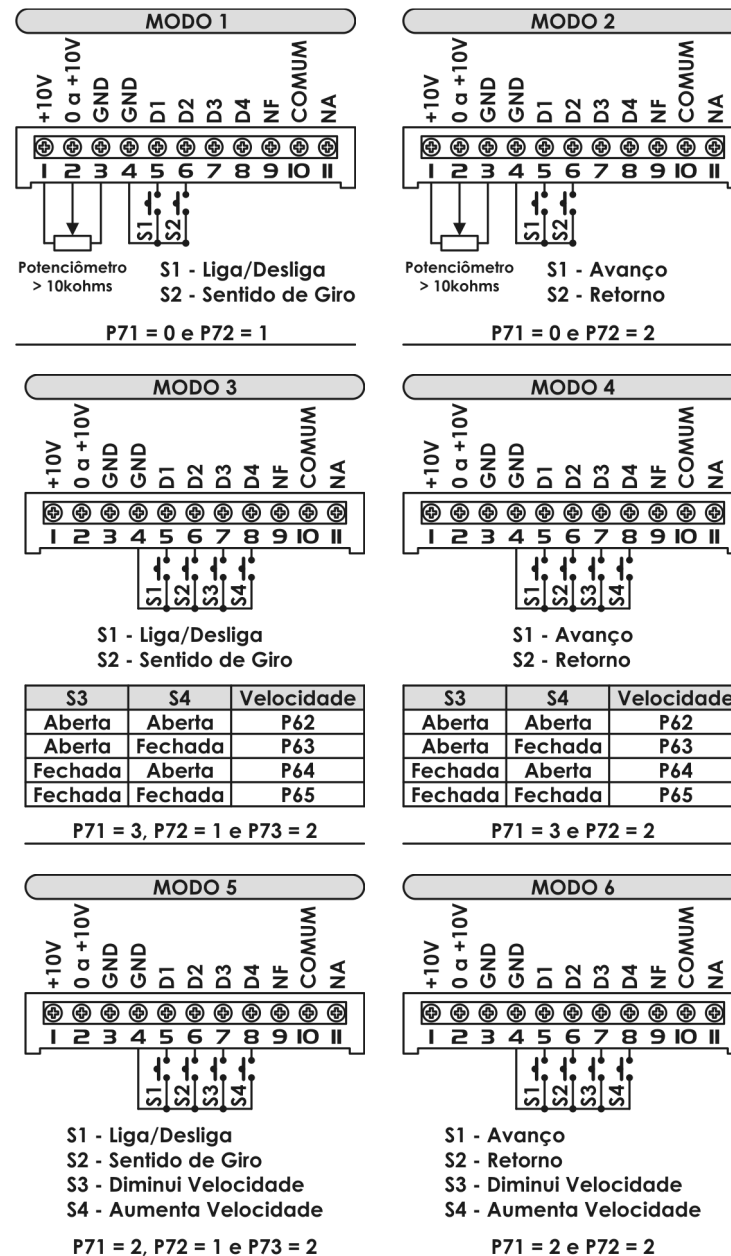
Figura 10-3 – Modos de Funcionamento Através dos Bornes de Controle
